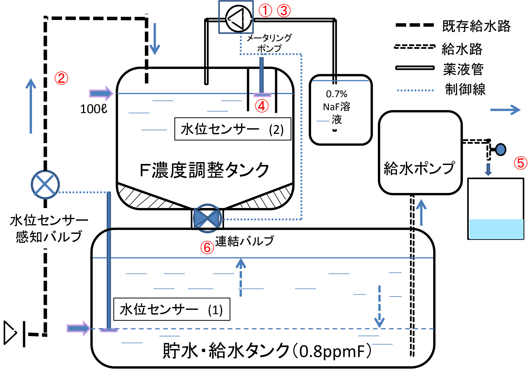
[ 施設フロリデーション設計図 ]
